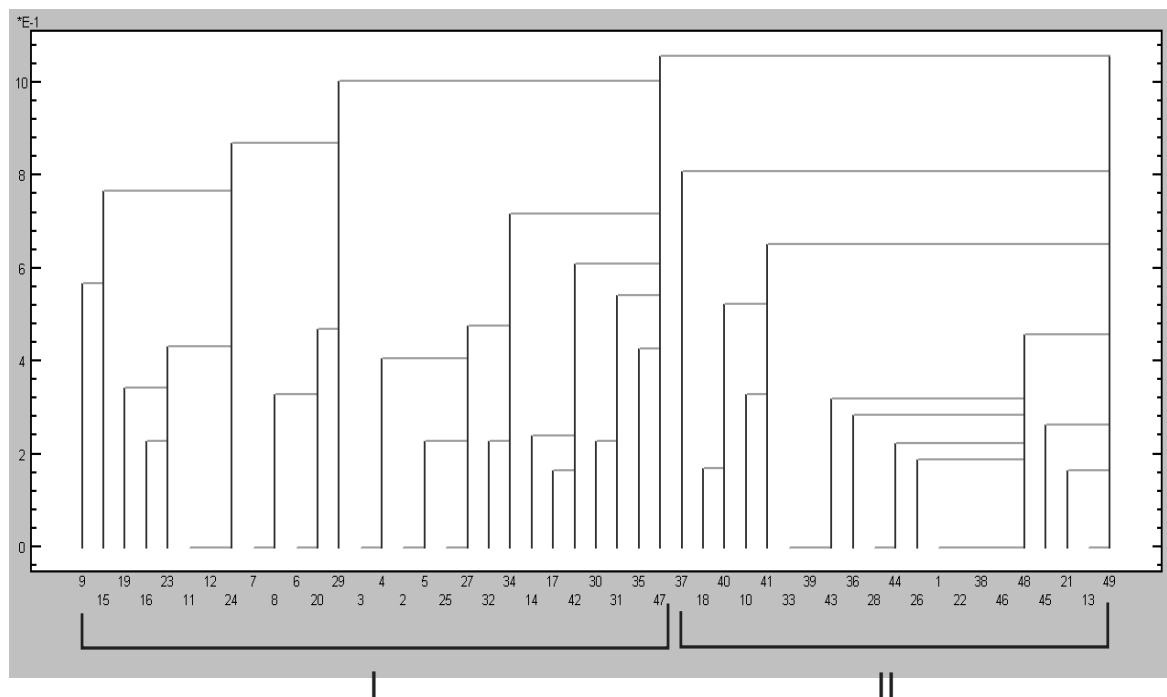
Рис. 2. Дендрограмма кластерных расстояний между инвазивными видами, построенная по данным их фитоценотической приуроченности
